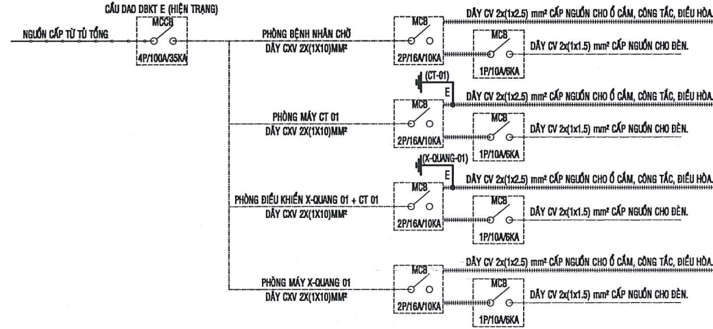
SƠ ĐỒ NGUYÊN LÝ PHÒNG ĐẶT MÁY X-QUANG 01 VÀ CT 01
