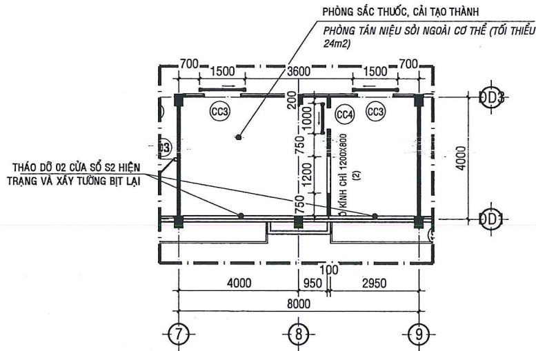
MẶT BẰNG CẢI TẠO PHÒNG ĐẶT MÁY TÁN SỎI NHIỆU NGOÀI CƠ THỂ TL:1/100 (DỰ ÁN MUA SẴM THIẾT BỊ Y TẾ CỦA BỆNH VIỆN ĐA KHOA TỈNH NĂM 2025)
