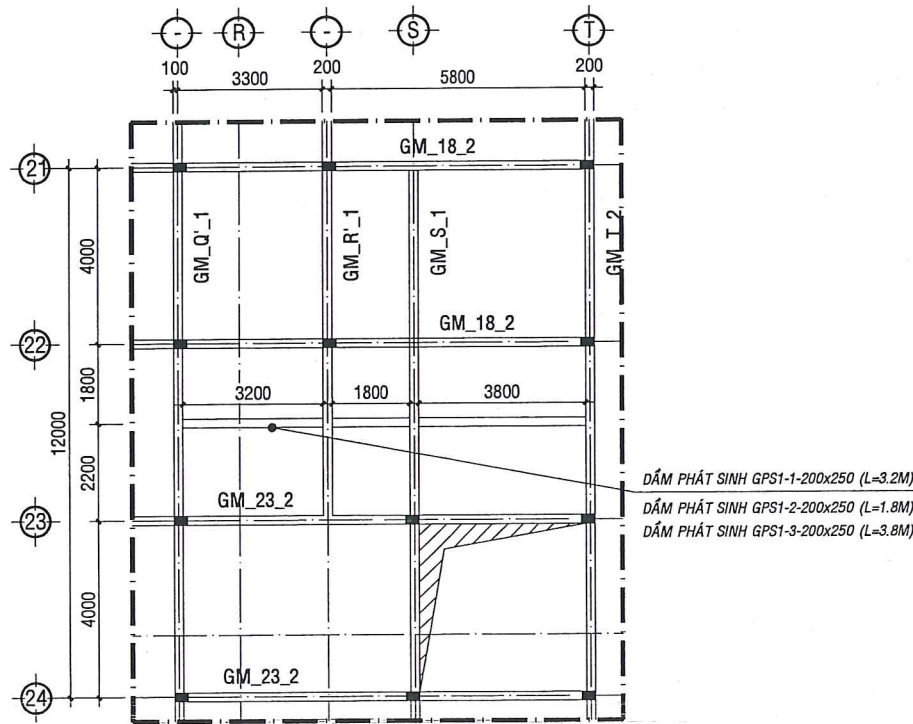
MẶT BẰNG DẦM PHÁT SINH PHÒNG ĐẶT MÁY X-QUANG 01 VÀ CT 01 TL:1/100
