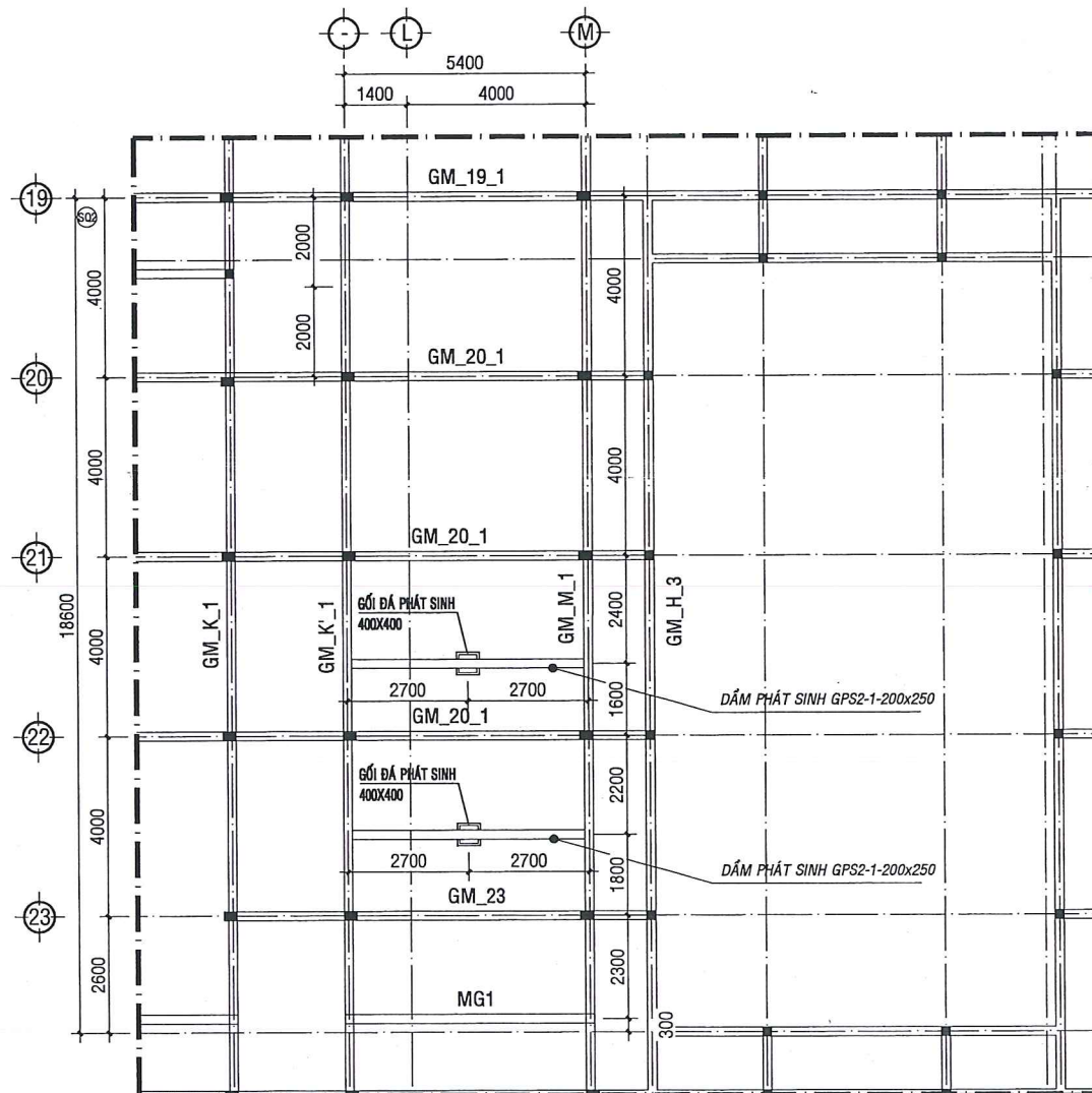
MẶT BẰNG DẦM PHÁT SINH PHÒNG ĐẶT MÁY X-QUANG 02 VÀ CT 02 TL:1/100
