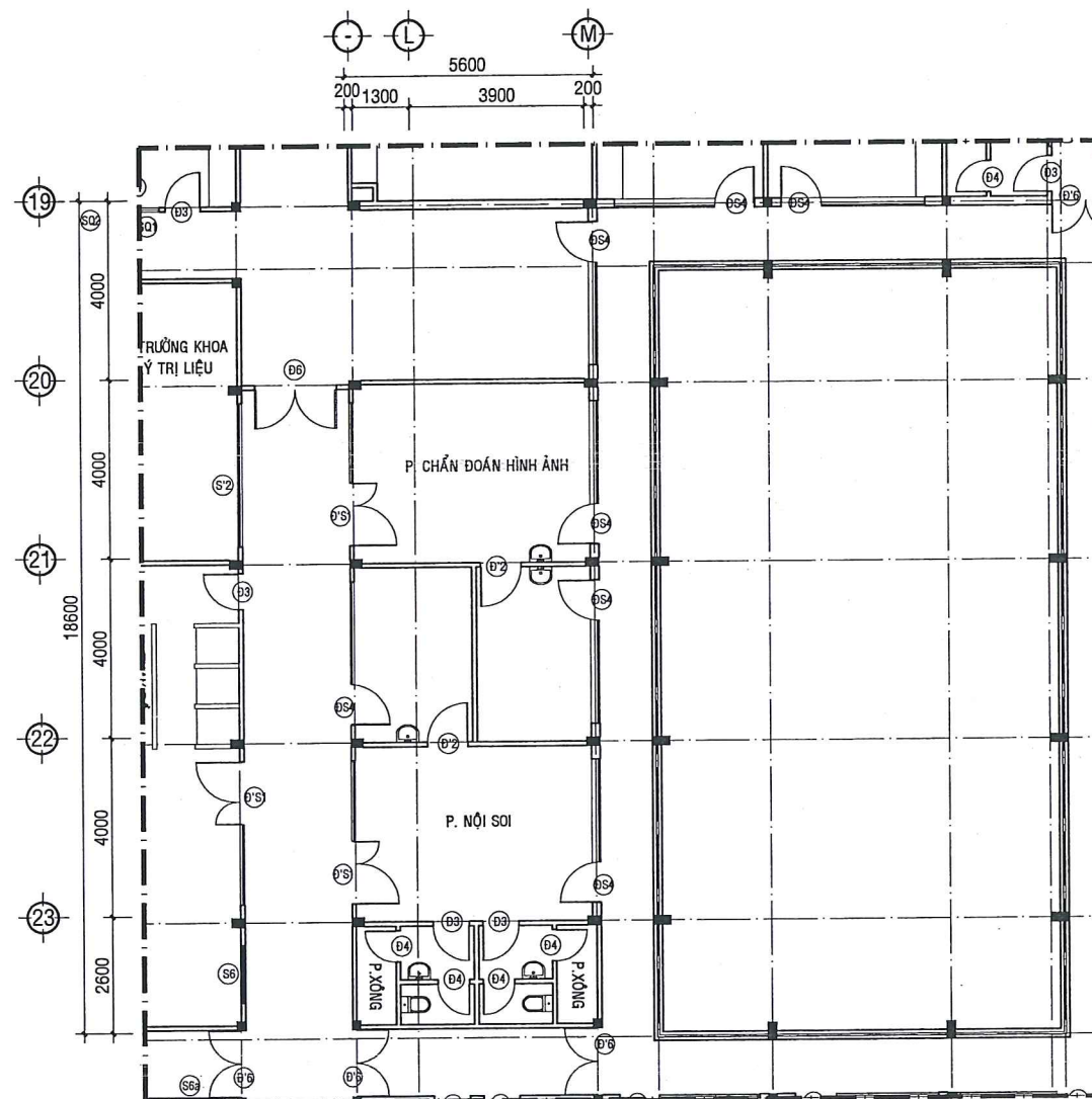
MẶT BẰNG HIỆN TRẠNG PHÒNG CHẨN ĐOÁN HÌNH ẢNH VÀ PHÒNG NỘI SOI TL:1/100 (KHỐI KỸ THUẬT NGHIỆP VỤ)
