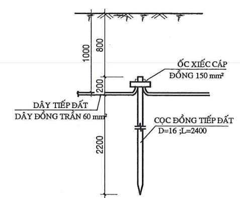
CHI TIẾT CỌC ĐỒNG TIẾP ĐẤT
