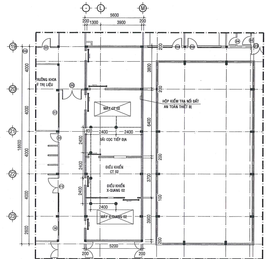
MẶT BẰNG CHỐNG SÉT PHÒNG ĐẶT MÁY X-QUANG 02 VÀ CT 02 TL:1/100
