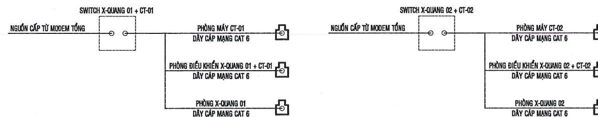
SƠ ĐỒ NGUYÊN LÝ CẤP MẠNG PHÒNG X-QUANG 01 + CT-01
