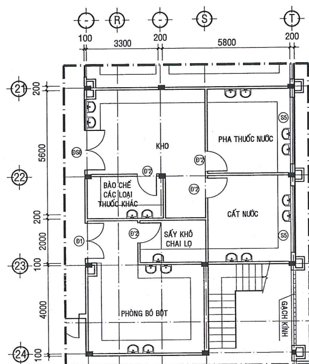
MẶT BẰNG HIỆN TRẠNG KHO DƯỢC VÀ PHÒNG BÓ BỘT TL:1/100 (KHỐI KỸ THUẬT NGHIỆP VỤ)
