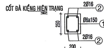
CHI TIẾT GPS2-1 - TL: 1/10 L= 5.6M, SL= 02 CK
