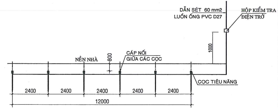
CHI TIẾT BÃI CỌC TIẾP ĐẤT
