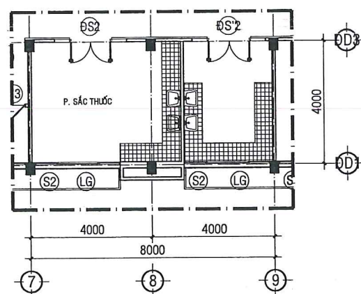
MẶT BẰNG HIỆN TRẠNG PHÒNG SẮC THUỐC TL:1/100 (KHỐI C3)
