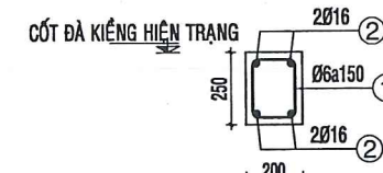
CHI TIẾT GPS1-3 - TL: 1/10 L= 4.2M, SL= 01 CK
