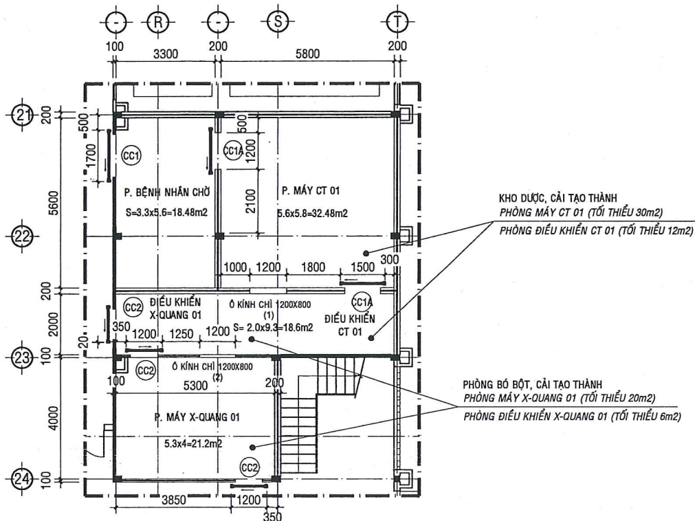
MẶT BẰNG CẢI TẠO PHÒNG ĐẶT MÁY X-QUANG 01 VÀ CT 01 TL:1/100 (DỰ ÁN MUA SẴM THIẾT BỊ Y TẾ CỦA BỆNH VIỆN ĐA KHOA TỈNH NĂM 2025)
