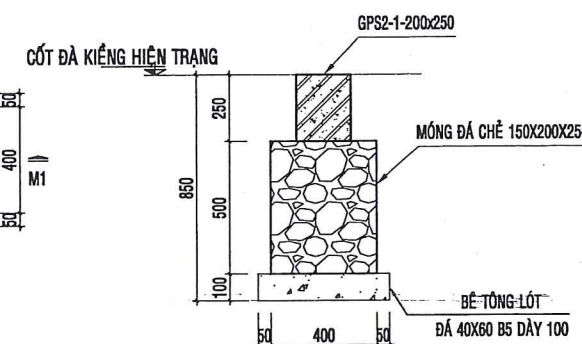
MẶT CẮT M1-M1 - TL: 1/25
