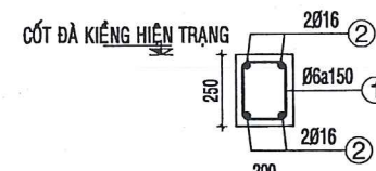
CHI TIẾT GPS1-2 - TL: 1/10 L= 2.2M, SL= 01 CK
