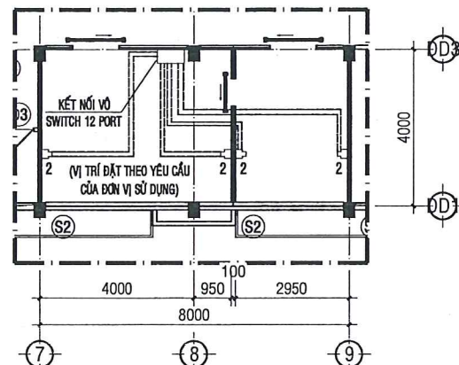
MẶT BẰNG CẤP MẠNG INTERNET PHÒNG ĐẶT MÁY TÁN SỎI NGOÀI CƠ THỂ TL:1/100
