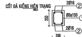
CHI TIẾT GPS1-1 - TL: 1/10 L= 3.6M, SL= 01 CK
