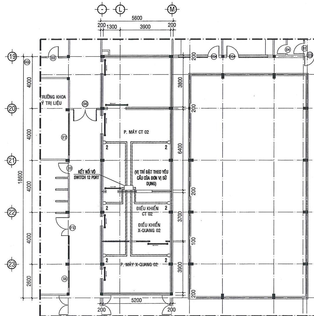
MẶT BẰNG CẤP MẠNG INTERNET PHÒNG ĐẶT MÁY X-QUANG 02 VÀ CT 02 TL:1/100
