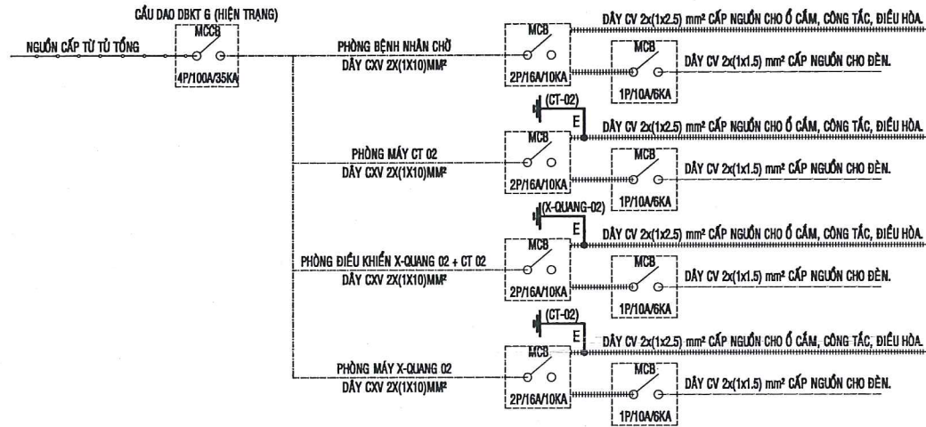
SƠ ĐỒ NGUYÊN LÝ PHÒNG ĐẶT MÁY X-QUANG 02 VÀ CT 02
