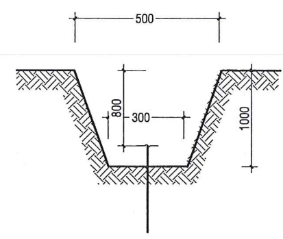
MẶT CẮT NGANG HỒ ĐÀO TIẾP ĐỊA
