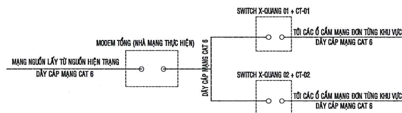
SƠ ĐỒ NGUYÊN LÝ CẤP MẠNG TỔNG KHỐI NGHIỆP VỤ
