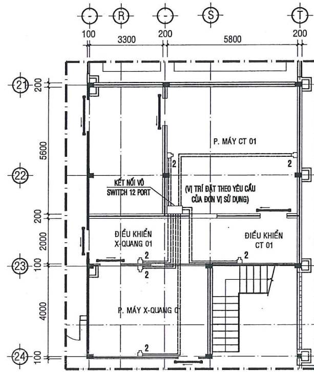
MẶT BẰNG CẤP MẠNG INTERNET PHÒNG ĐẶT MÁY X-QUANG 01 VÀ CT 01 TL:1/100
