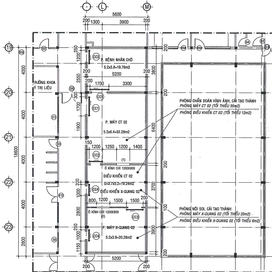
MẶT BẰNG CẢI TẠO PHÒNG ĐẶT MÁY X-QUANG 02 VÀ CT 02 TL:1/100 (DỰ ÁN MUA SẴM THIẾT BỊ Y TẾ CỦA BỆNH VIỆN ĐA KHOA TỈNH NĂM 2025)
